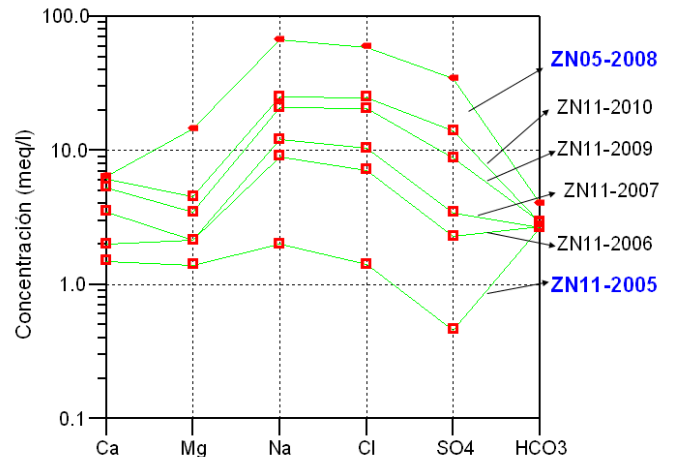
Figura 4. Diagramas de Schoeller del Pozo ZN11
