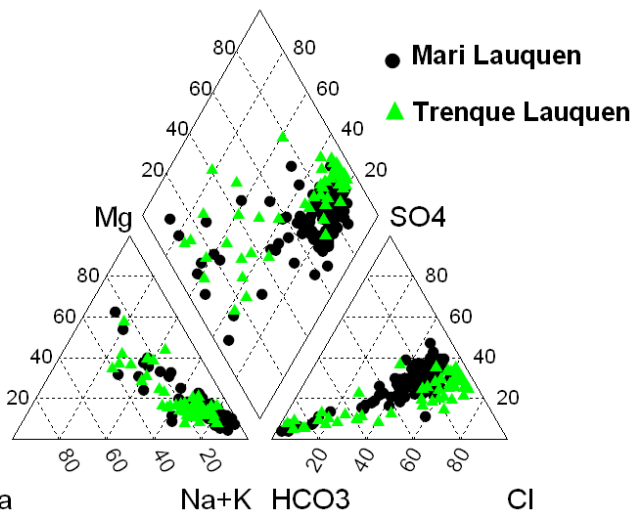
Figura 2. Diagrama de Piper de pozos de Zona Norte de Trenque Lauquen y de Mari Lauquen (2005-2010)
