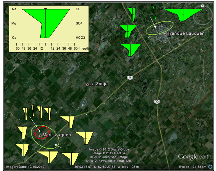
Figura 3. Distribución espacial de Diagramas de Stiff, para el año 2010
