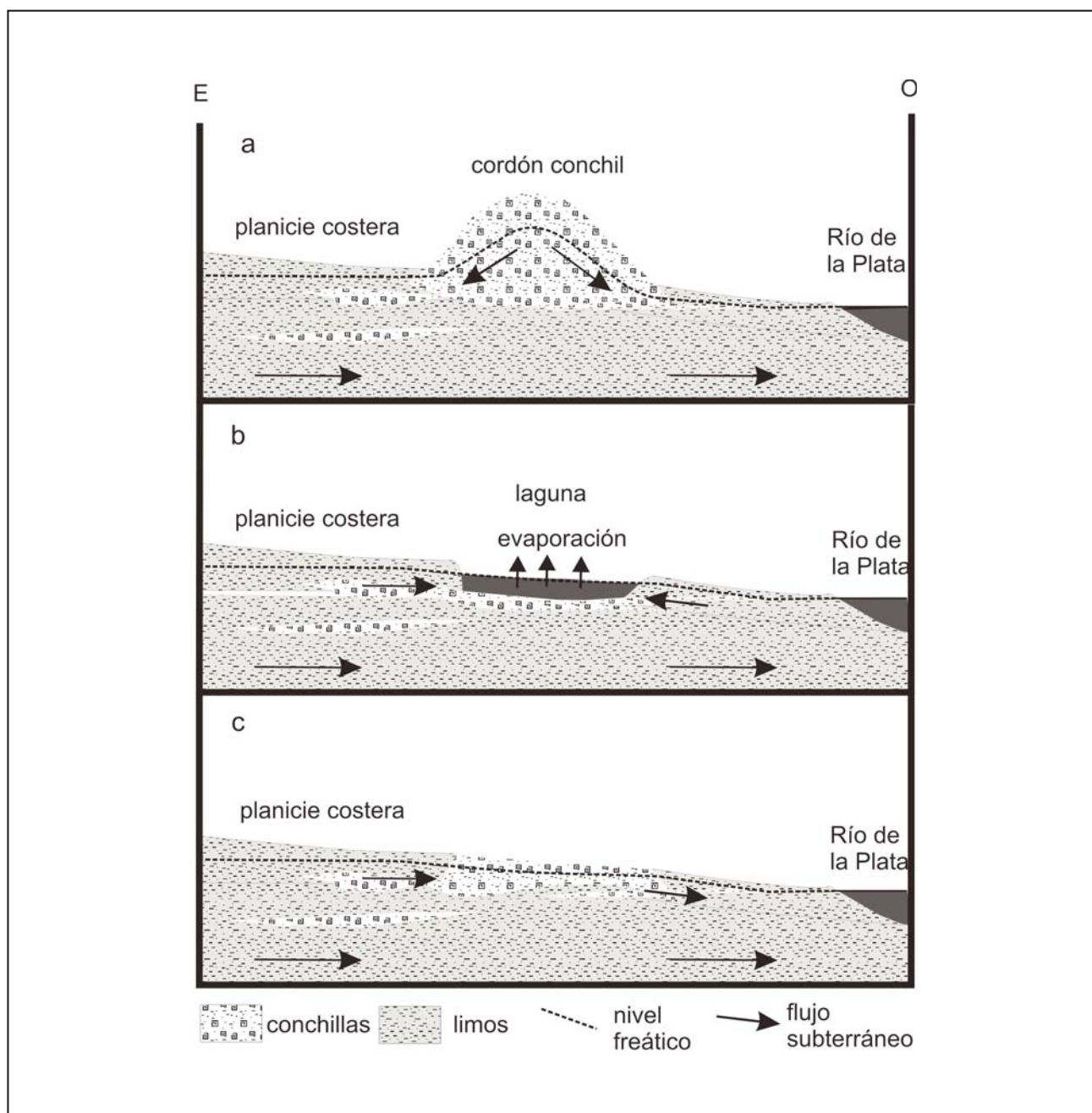
Figura 2. Esquemas de posición del nivel freático y flujo subterráneo en condiciones naturales y luego de la explotación.
