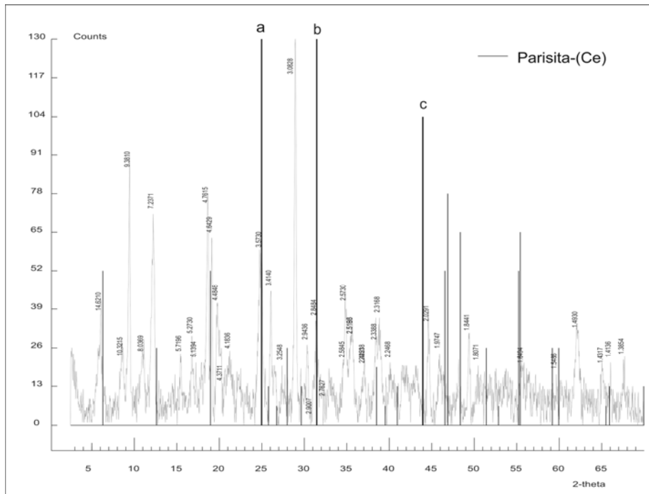
Fig. 5: difractograma de rayos X de la muestra 11.048 (pelita roja masiva) con picos representativos de la Parisita-(Ce); realizado con Xpovder. Los picos principales a, b y c corresponden a los espaciados 3.565, 2.838 y 2.060 respectivamente.
