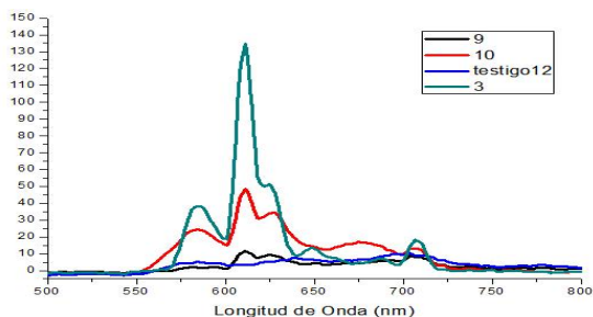
Fig 4: Espectros obtenidos para el caso de HPV6 perianal.
