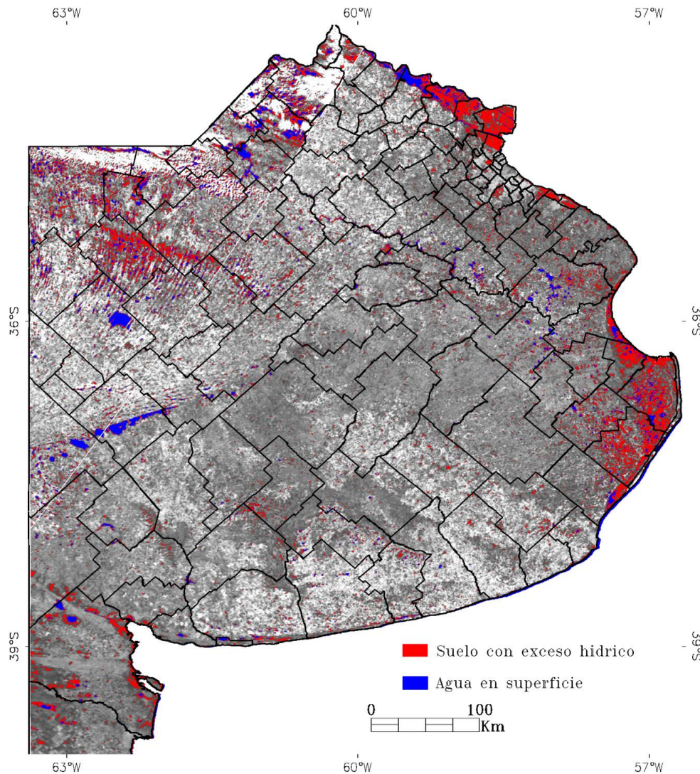
Imagen MODIS/Aqua, 500 m de resolución espacial del 23-ago-2016, muestra el área con exceso hídrico en superficie.
