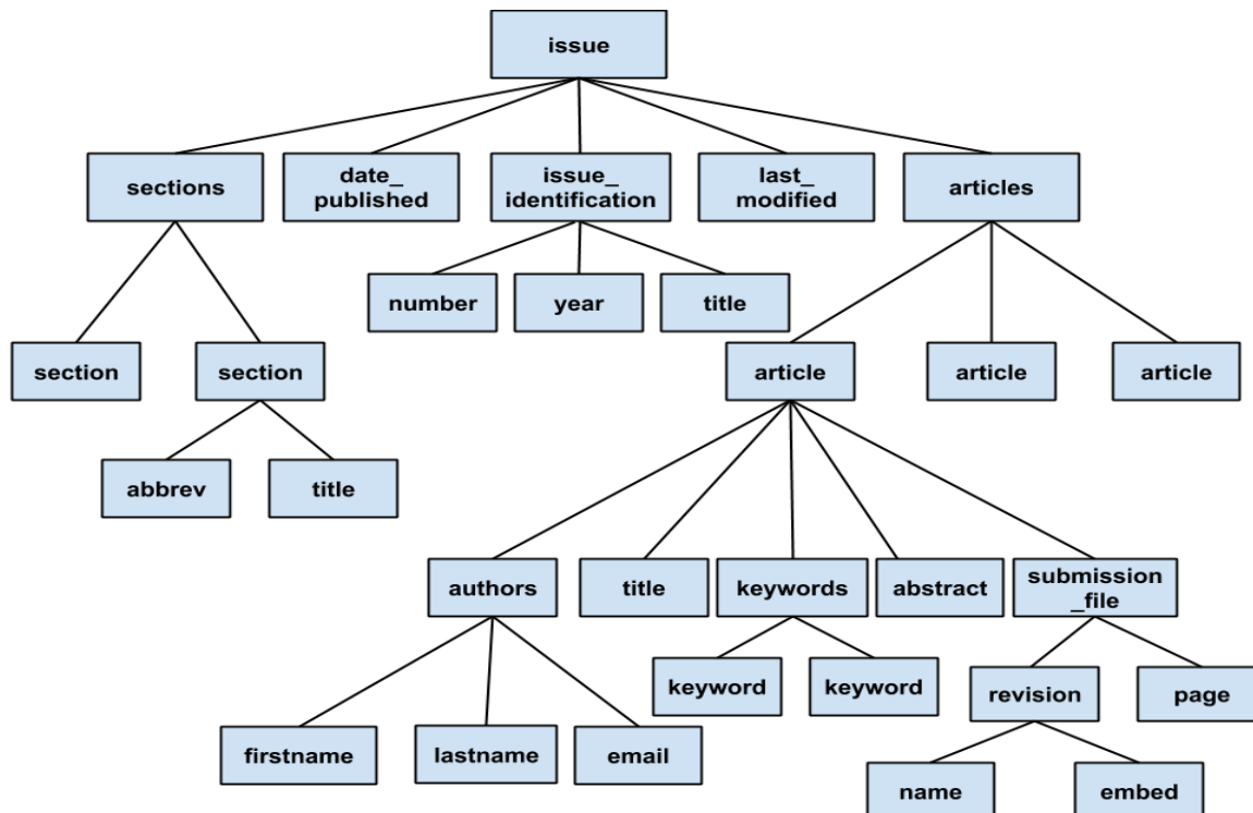
Imagen 5: Estructura jerárquica del XML nativo.
