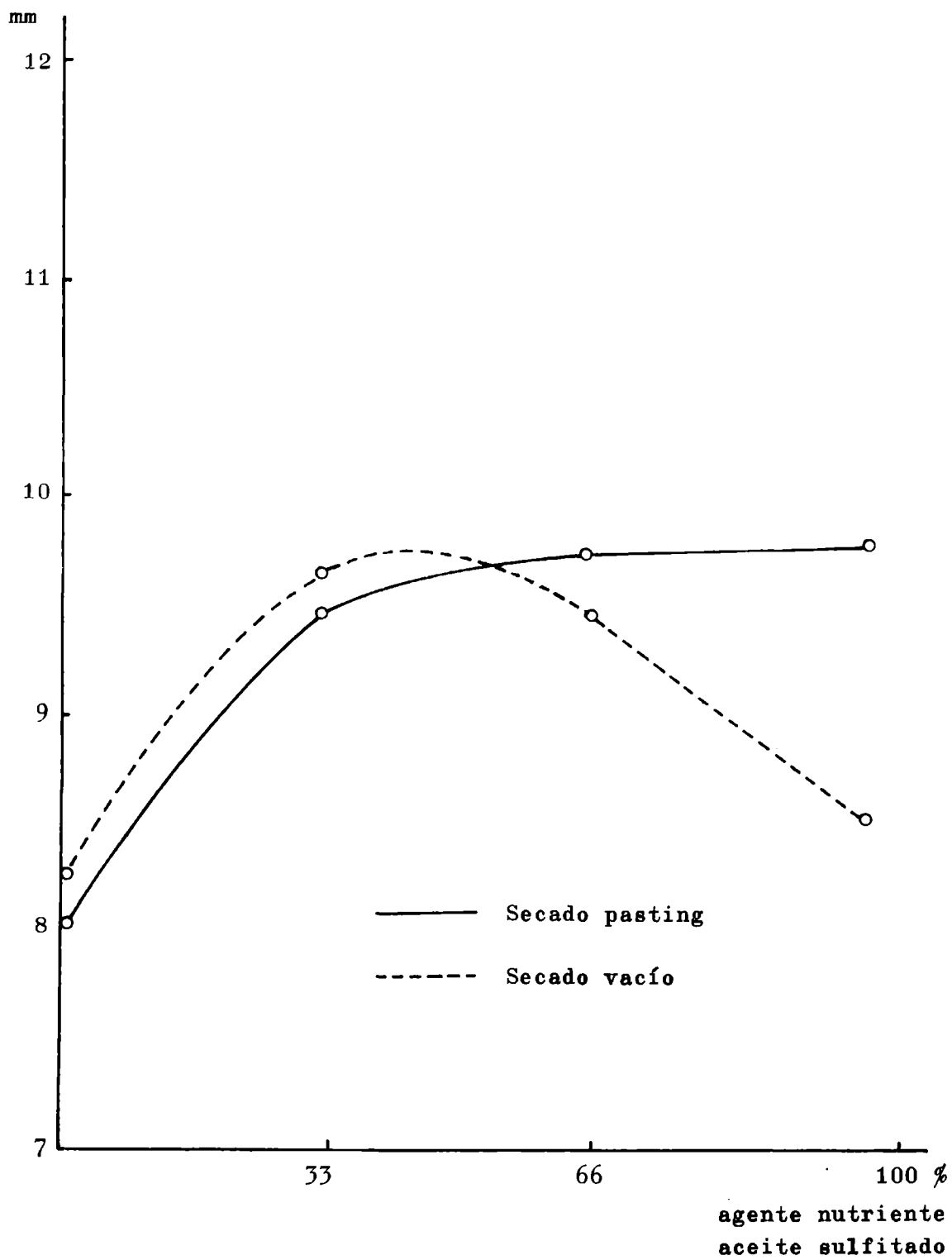
Fig. 2.- Distensión a la rotura de la flor (antes de desflovar)
