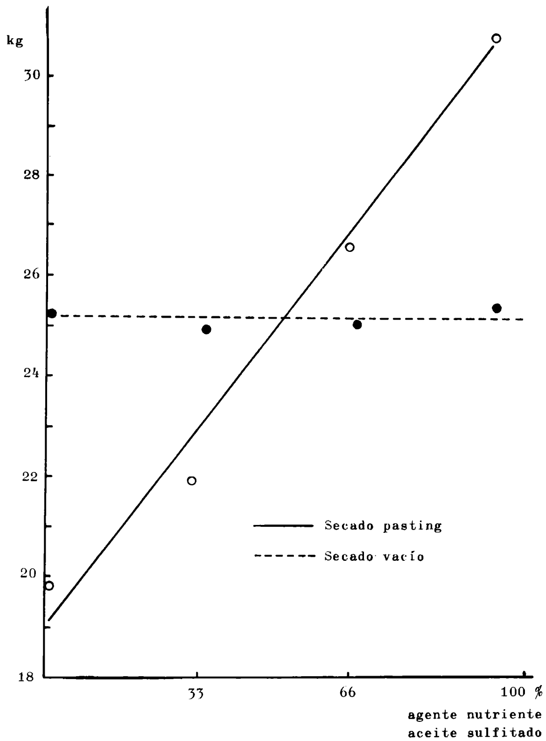
Fig. 1.- Resistencia al desgarramiento (antes de desflorar)
