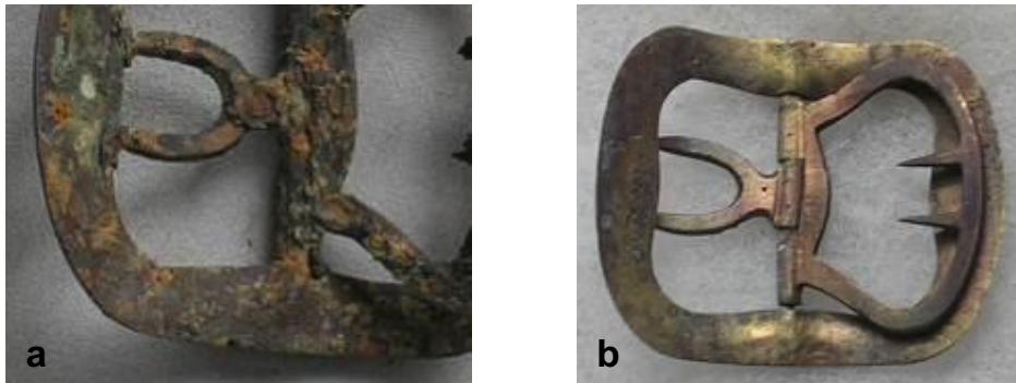
Figura 12. Limpieza con láser realizada a una hebilla a) antes de la limpieza. b) Después de la limpieza.
