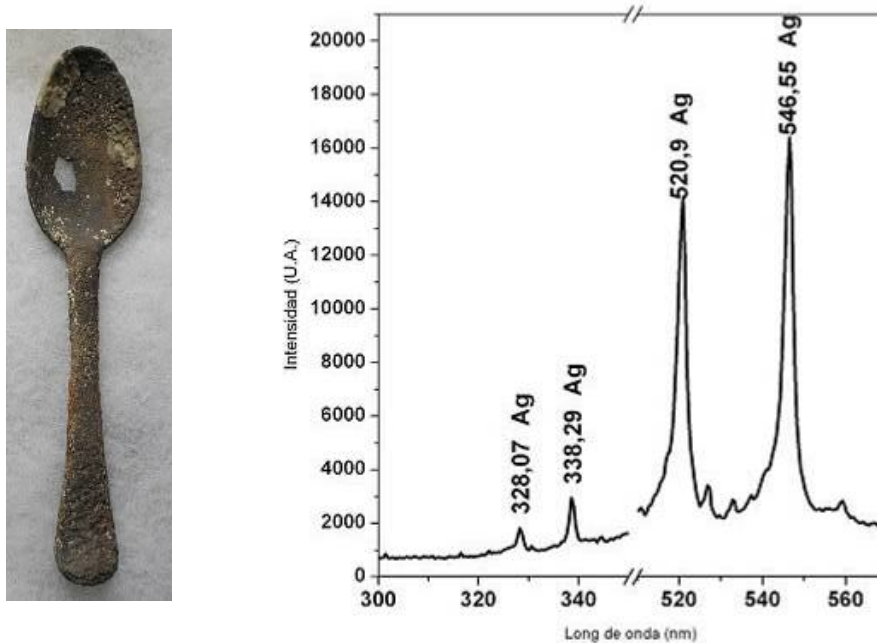
Figura 3. Cuchara N° 60 y espectro con líneas características del elemento constitutivo. Material: Plata
