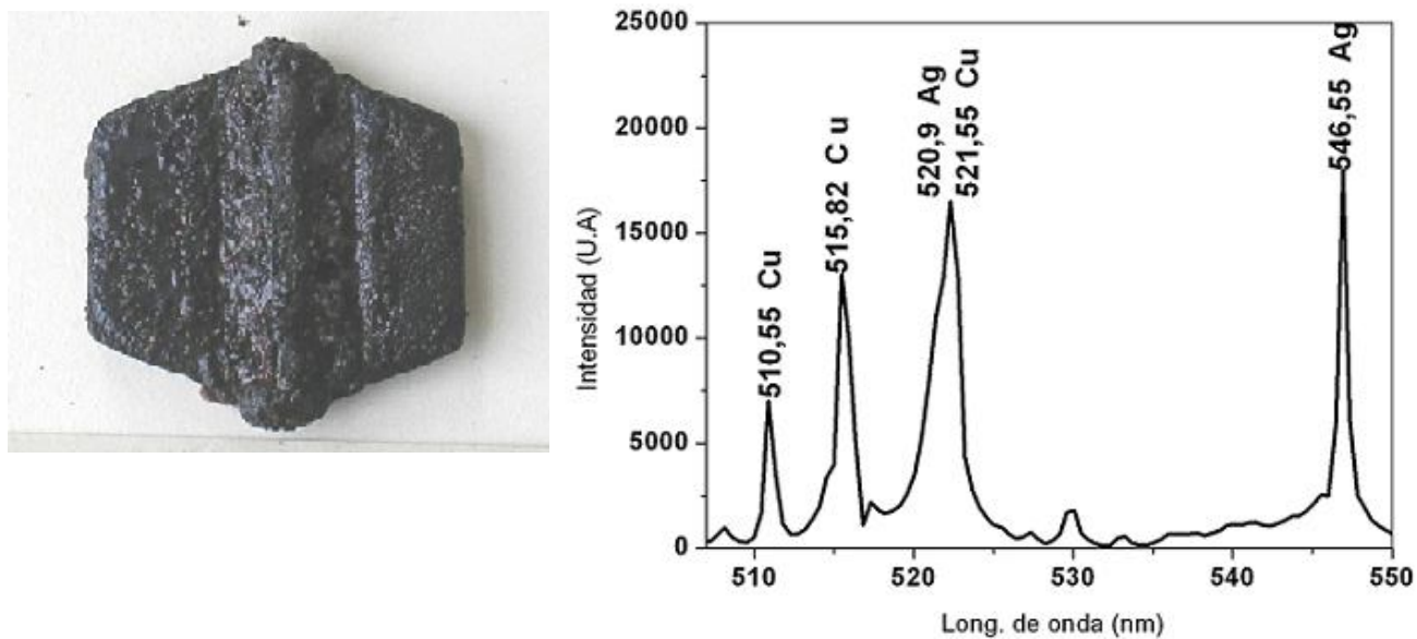
Figura 4. Bisagra y Espectro LIBS correspondiente. Material: cobre y plata
